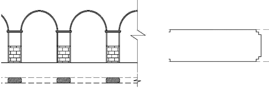
شكل (25) مسقط أفقي لإحدى الاكتاف البنائية بجامع عمرو واجهة للعقود النصف دائرية التي تنتهي بها الاكتاف البنائية 14 .
