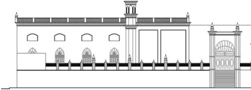
شكل (30) الواجهة الرئيسية لجامع عمر وواضح فيها مدى تنوع عناصرها المعمارية.
