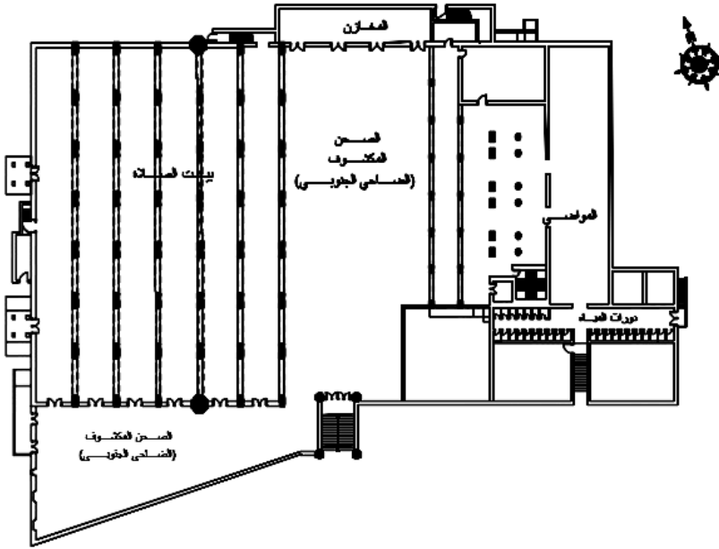
شكل (23) المسقط الافقي لجامع عمر 13 .
