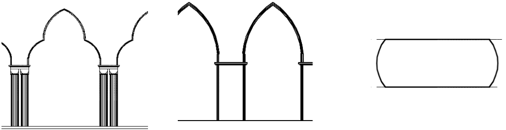
شكل (6) مسقط أفقي وواجهة لأشكال الاكشاف البنائية بجامع البلاد والتي تنهي بعقود مدببة وعقود ذات المراكز الثلاثة 3 .
